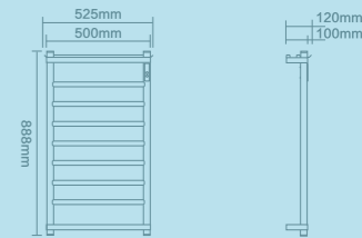
正面线图 / Front line diagram 侧面线图 / Side line drawing
