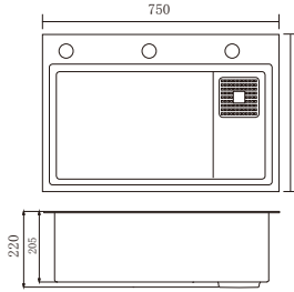
型号: ZP7545DH 规格: 750x450x220mm 开孔尺寸: 720x420mm
