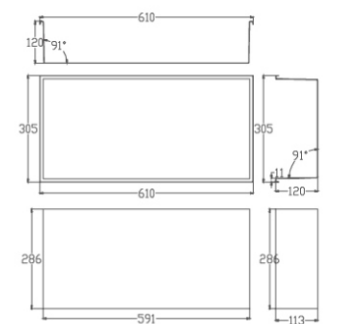
产品尺寸图:
