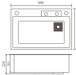
型号: ZP6846FYH 规格: 680x460x220mm 开孔尺寸: 650x430mm
