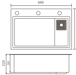
型号: ZP6845DH 规格: 680x450x220mm 开孔尺寸: 650x420mm
