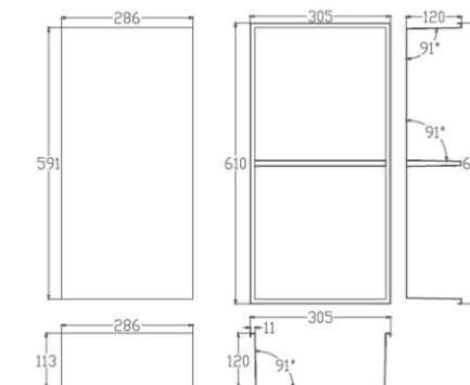
产品尺寸图：
