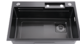
型号: ZP6846FYH 规格: 680x460x220mm 开孔尺寸: 650x430mm
