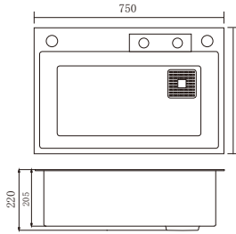
型号: ZP7546FYH 规格: 750x460x220mm 开孔尺寸: 720x430mm
